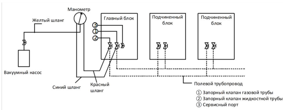
Рисунок 3-5.15. Вакуумная сушка
