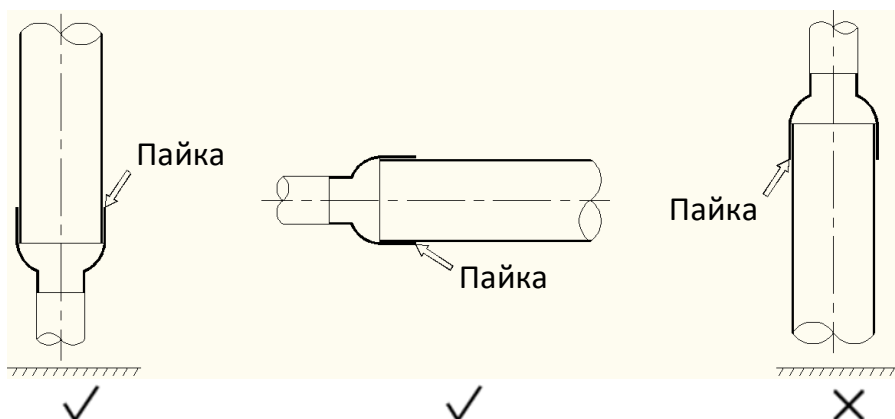
Рисунок 3-5.6. Ориентация трубопровода при пайке
