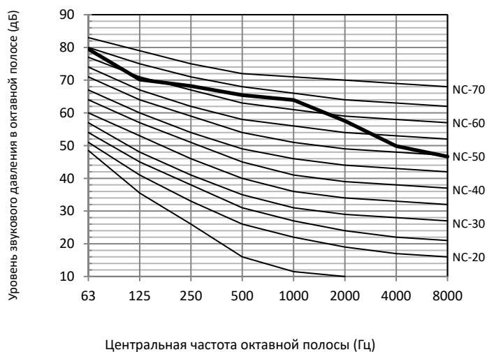
Рисунок 2-10.16. Уровень октавной полосы модели 36 л. с.
