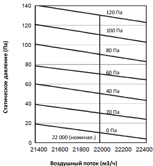
Рисунок 3-3.11. Производительность вентилятора блоков мощностью 20–26 л. с.
