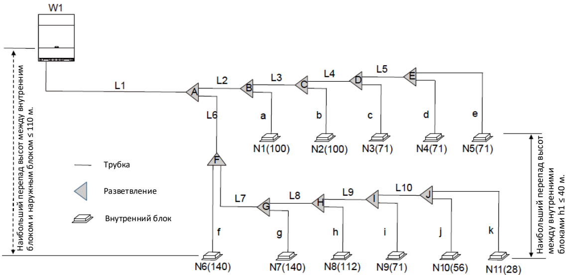
Рисунок 3-4.4. Пример выбора трубопровода хладагента
