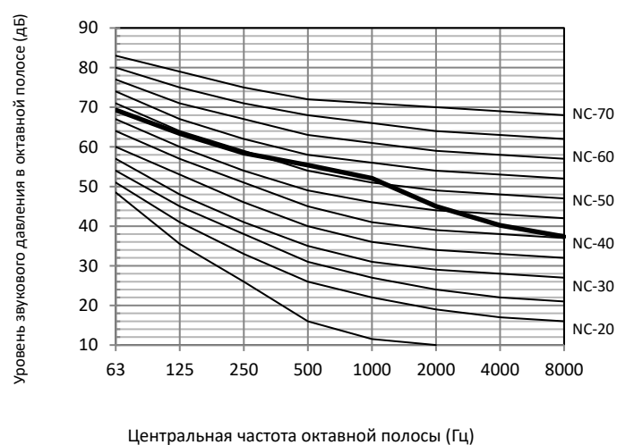
Рисунок 2-10.5. Уровень октавной полосы модели 14 л. с.
