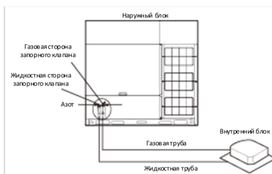
Рисунок 3-5.14. Испытание на газонепроницаемость
