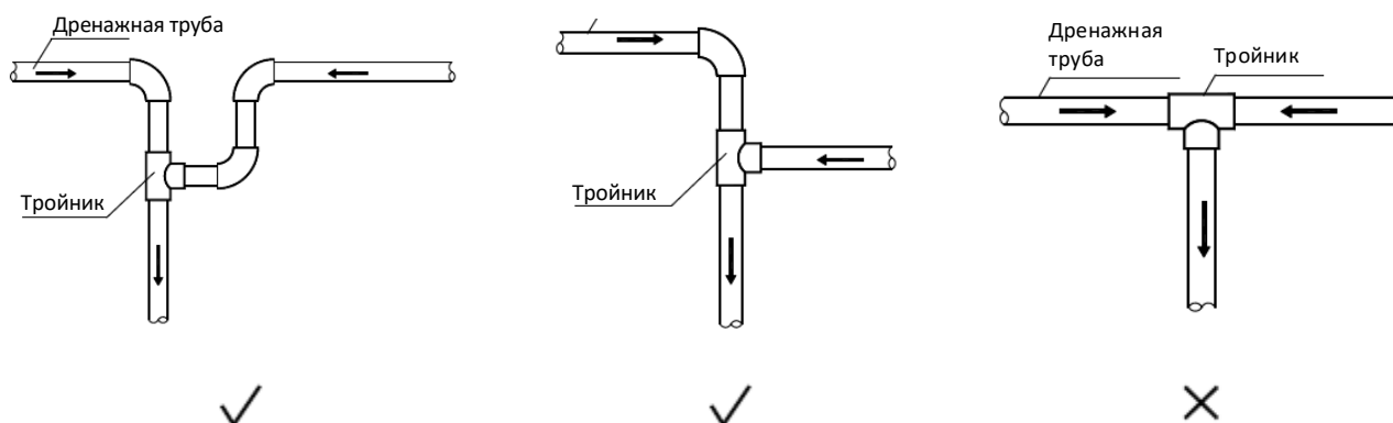
Рисунок 3-6.2. Соединения дренажных трубопроводов — правильные и неправильные конфигурации
