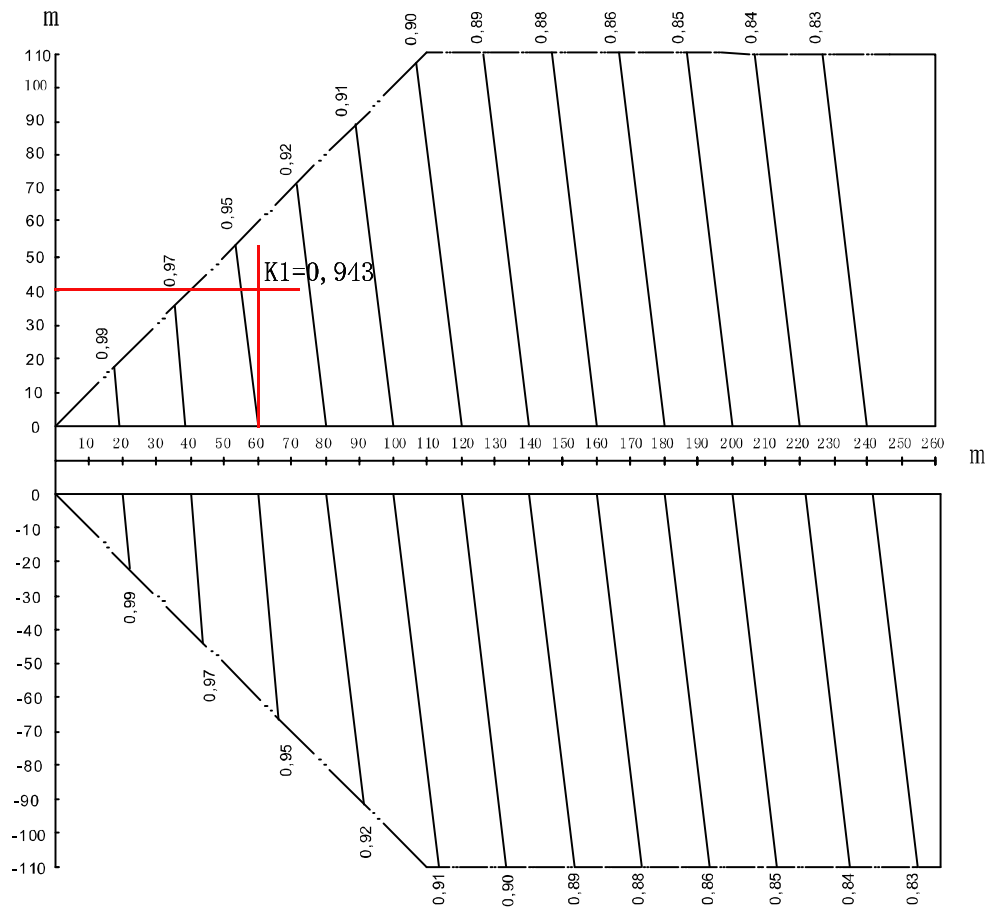
Рисунок 1-5.3. Скорость изменения мощности охлаждения V8i
