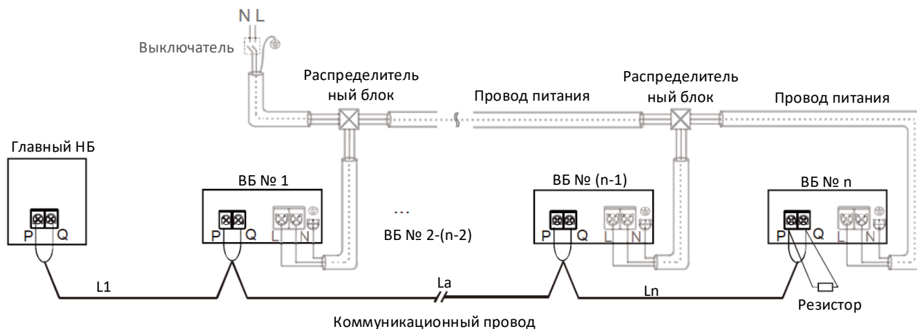
Рисунок 3-9.8. Конфигурация коммуникационной проводки P Q – единое питание ВБ
