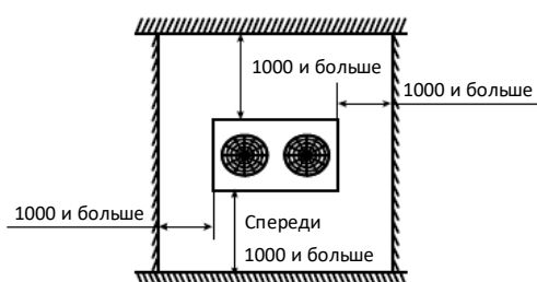
Рисунок 3-2.1. Установка одноканального блока (ед. изм.: мм)
