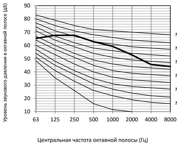
Рисунок 2-10.12. Уровень октавной полосы модели 28 л. с.
