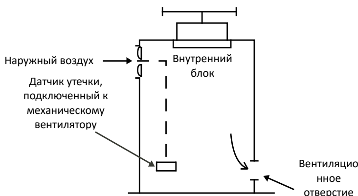
Рисунок 3-4.7. Механический вентилятор, управляемый датчиком утечки хладагента
