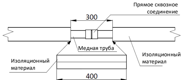
Рисунок 3-7.1. Установка изоляции соединений (ед. изм.: мм)
