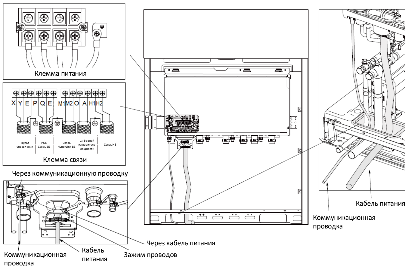
Рисунок 3-9.1. Схема электропроводки
