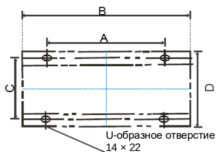
Рисунок 3-2.5. Расположение анкерных болтов
