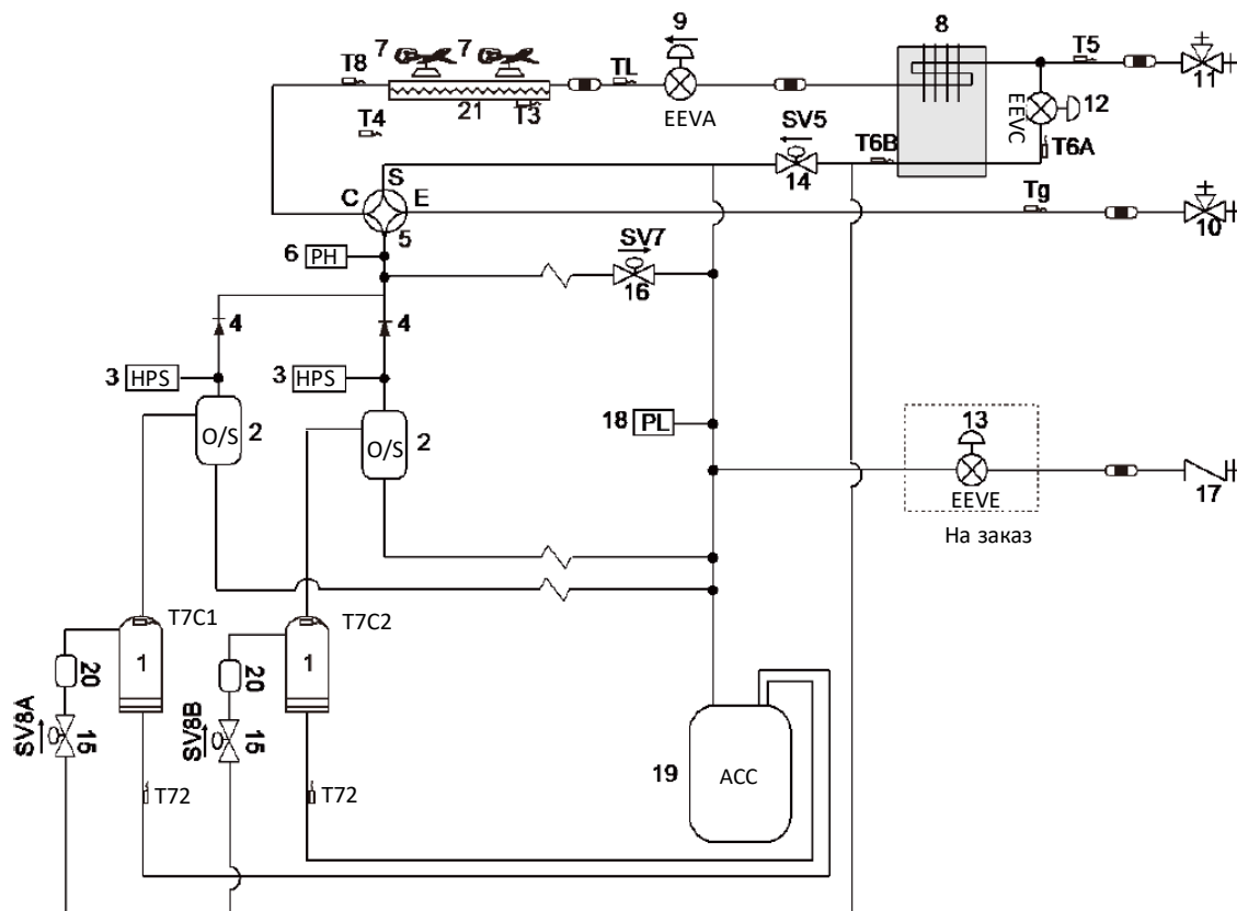
Рисунок 2-4.2. Схема трубопровода модели 20–26 л. с.
