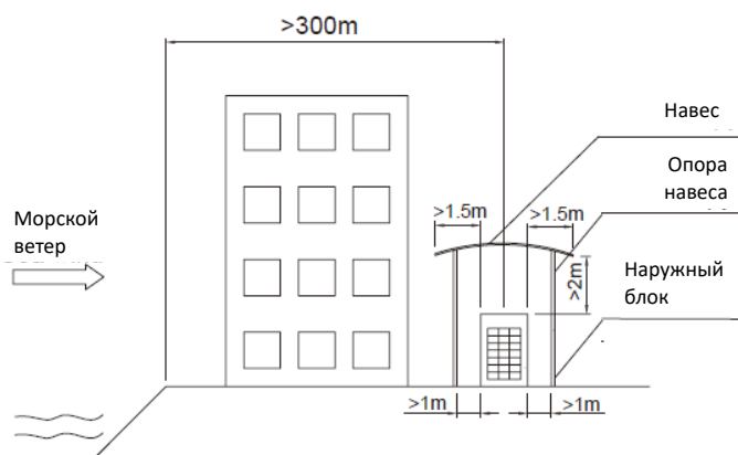
Рисунок 3-10.2. Установка на открытом воздухе под навесом
