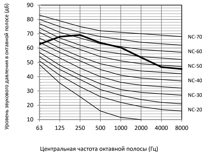
Рисунок 2-10.13. Уровень октавной полосы модели 30 л. с.
