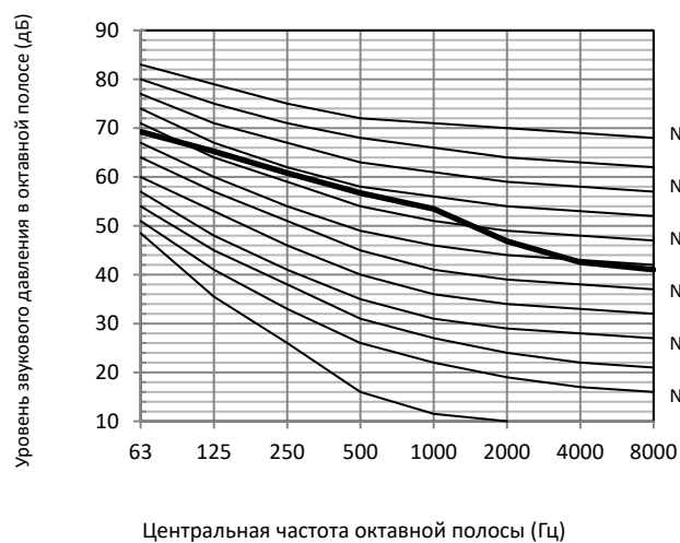
Рисунок 2-10.6. Уровень октавной полосы модели 16 л. с.
