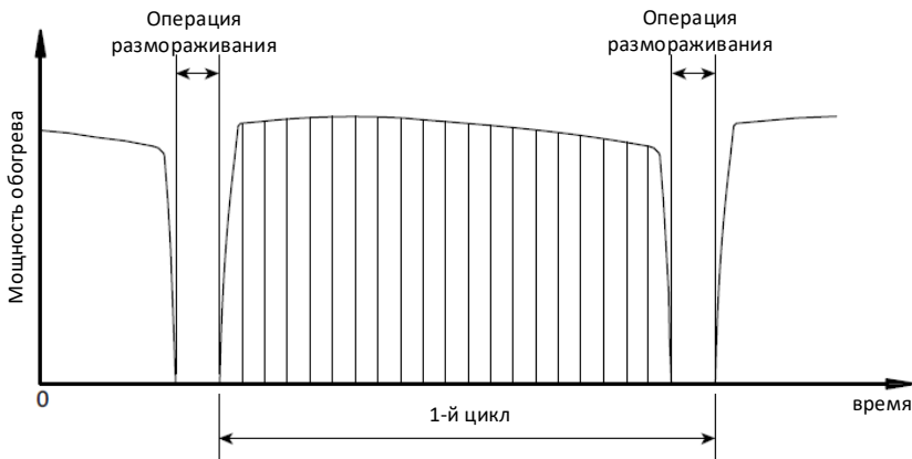
Рисунок 2-8.3. Цикл размораживания
