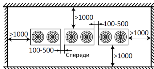
Рисунок 2-3.2. Однорядная установка (ед. изм.: мм)
