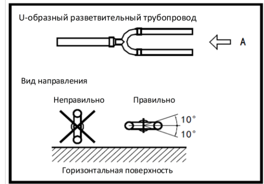
Рисунок 3-5.8. Ориентация разветвителей
