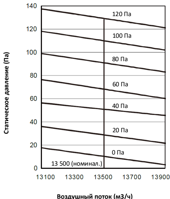
Рисунок 3-3.9. Производительность вентилятора блоков мощностью 8–14 л. с.
