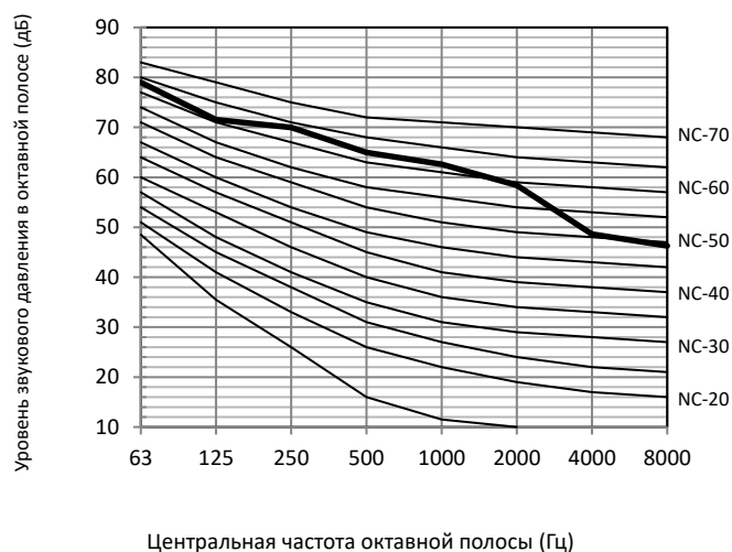
Рисунок 2-10.16. Уровень октавной полосы модели 36 л. с.
