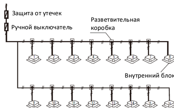
Рисунок 3-9.3. Унифицированная проводка питания внутреннего блока
