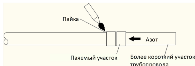
Рисунок 3-5.5. Пропускание азота с более короткой стороны во время пайки
