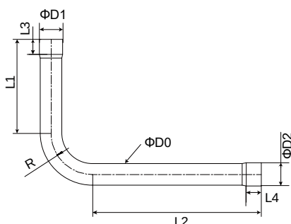
Рисунок 2-11.1. Размер Г-образного патрубка
