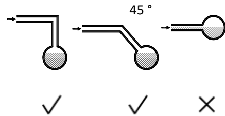
Рисунок 3-6.3. Дренажный трубопровод ответвления, соединяющийся с магистральным дренажным трубопроводом
