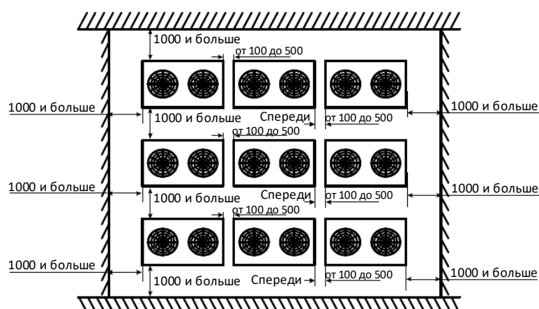
Рисунок 3-2.3. Многорядная установка (ед. изм.: мм)
