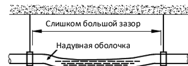
Рисунок 3-6.4. Влияние недостаточной опоры дренажного трубопровода
