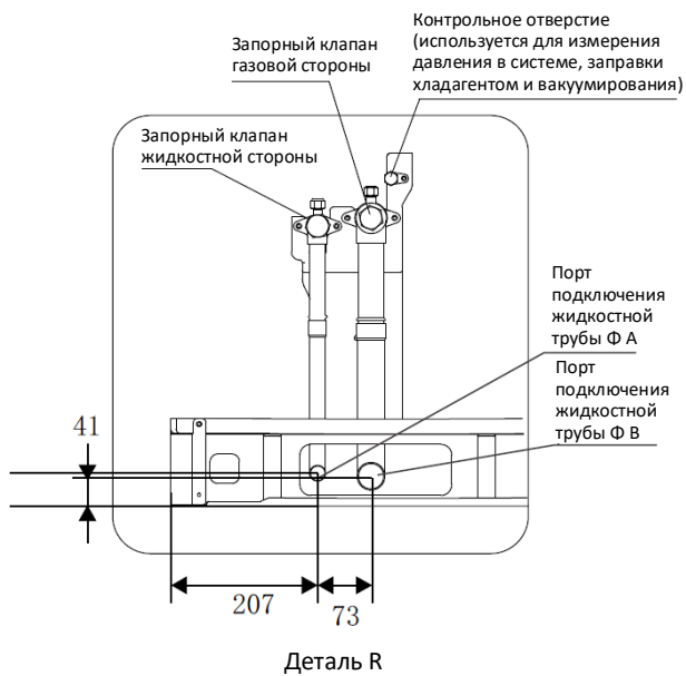
Рисунок 2-2.4. Деталь R (ед. изм.: мм)
