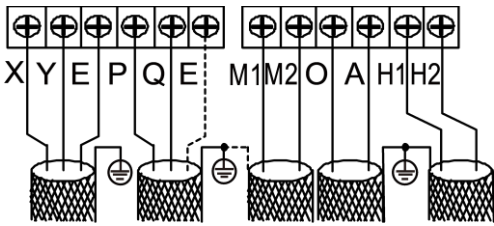
Рисунок 3-9.9. Коммуникационные клеммы главного наружного блока
