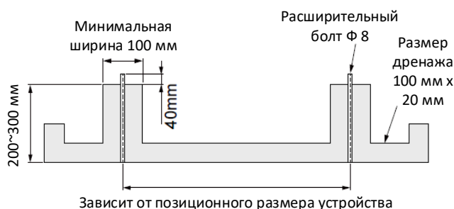
Рисунок 3-2.4. Типовой проект конструкции бетонного основания наружного блока (ед. изм.: мм)
