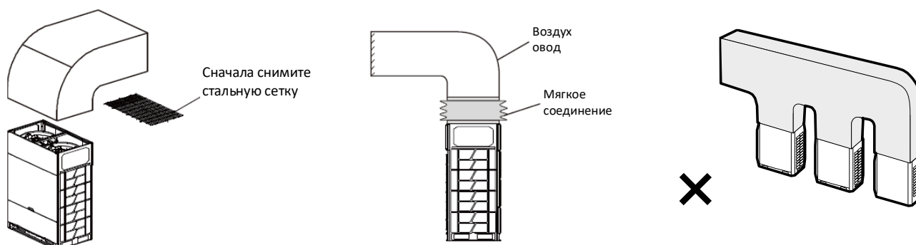
Рисунок 3-3.2. Требования к воздуховодам
