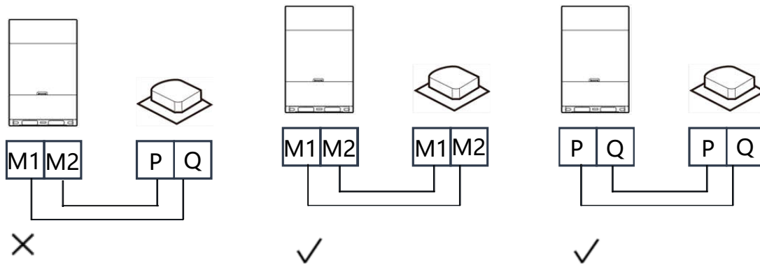
Рисунок 3-9.5. Коммуникационная проводка
