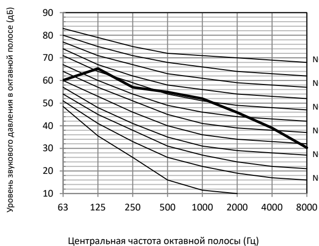
Рисунок 2-10.4. Уровень октавной полосы модели 12 л. с.
