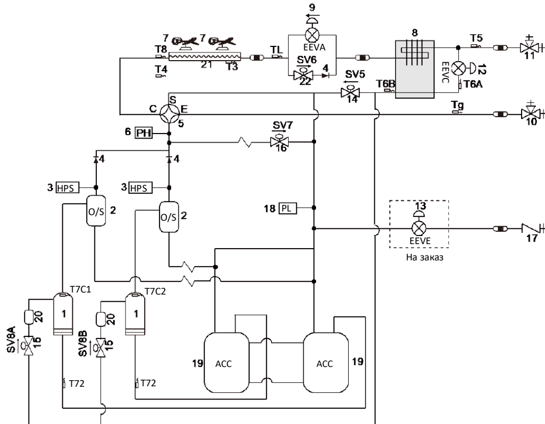
Рисунок 2-4.3. Схема трубопровода модели 28–36 л. с.
