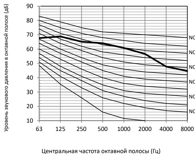
Рисунок 2-10.16. Уровень октавной полосы модели 36 л. с.
