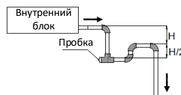
Рисунок 3-6.6. Сифоны дренажных трубопроводов
