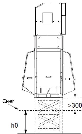
Рисунок 3-3.14. Защита наружного блока от снега
