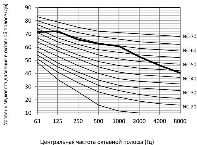
Рисунок 2-10.7. Уровень октавной полосы модели 18 л. с.
