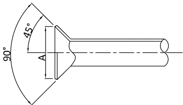
Рисунок 3-5.2. Развальцованное отверстие
