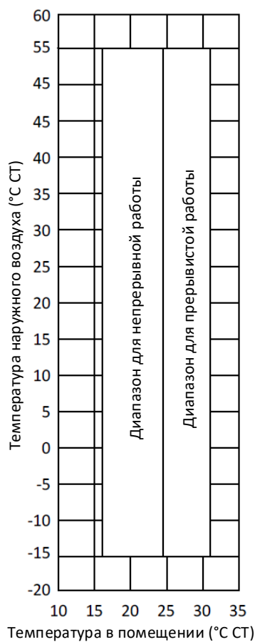
Рисунок 2-9.1. Рабочие пределы охлаждения
