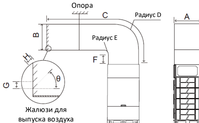
Рисунок 3-3.3. Продольные воздуховоды (ед. изм.: мм)
