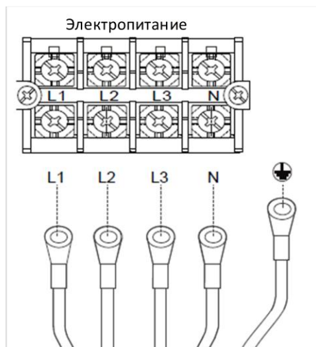
Рисунок 3-9.4. Клеммы 3-фазного питания наружного блока
