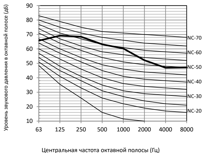
Рисунок 2-10.11: Уровень октавной полосы модели 26 л.с.
