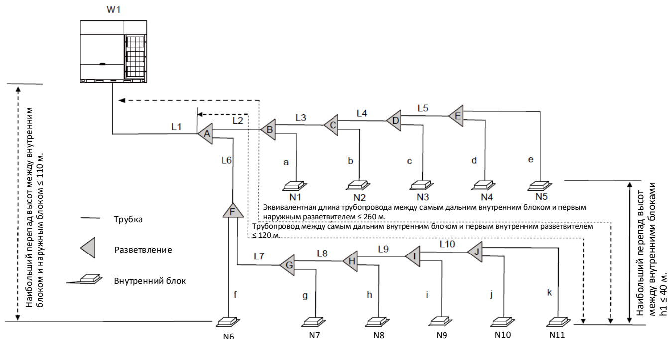
Рисунок 3-4.2. Допустимые значения длины трубопроводов хладагента и перепада высот
