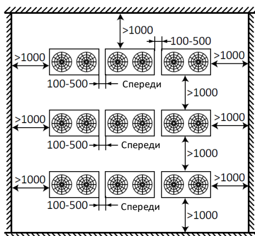
Рисунок 2-3.3. Многорядная установка (ед. изм.: мм)
