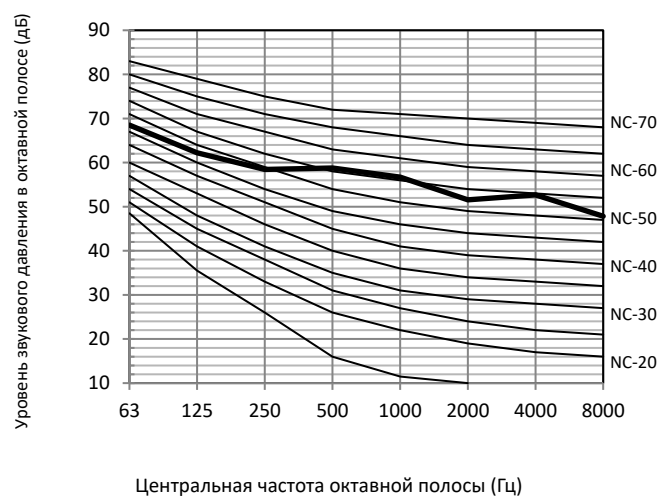
Рисунок 2-10.7. Уровень октавной полосы модели 18 л. с.
