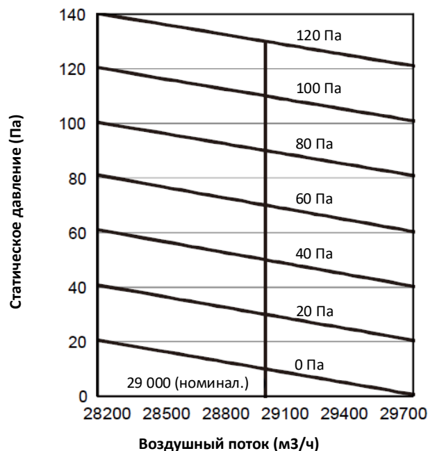
Рисунок 3-3.12. Производительность вентилятора блоков мощностью 28–36 л. с.
