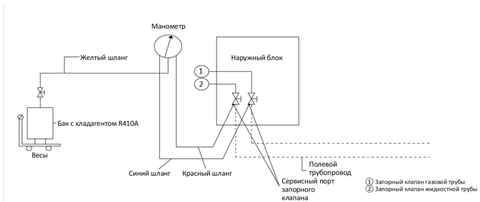
Рисунок 3-8.1. Заправка хладагентом
