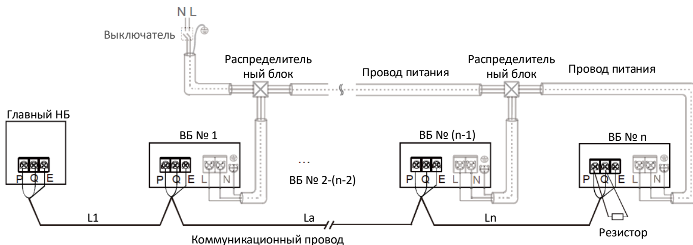
Рисунок 3-9.7. Конфигурация коммуникационной проводки P Q E – единое питание ВБ
