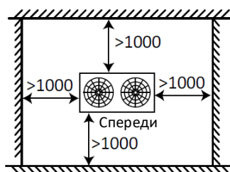
Рисунок 2-3.1. Установка одноканального блока (ед. изм.: мм)
