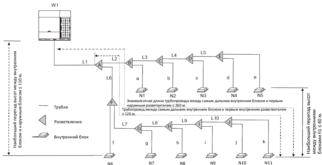
Рисунок 3-4.3. Выбор диаметров трубопроводов
