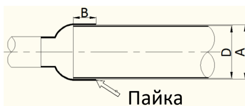
Рисунок 3-5.7. Перекрытие трубопроводов и зазор для паяных соединений
