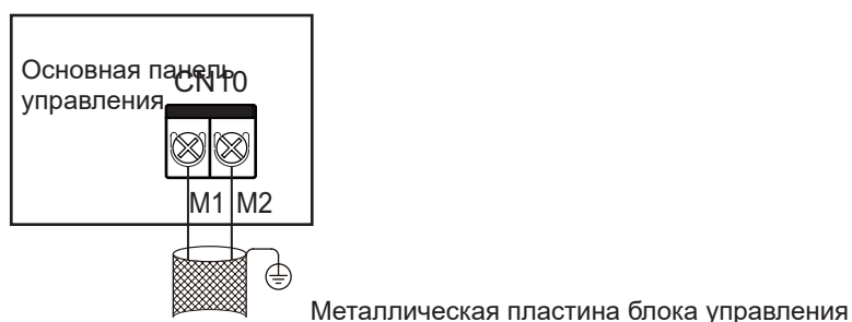
Подключение к наружному блоку M1M2 (MDV_Link)
