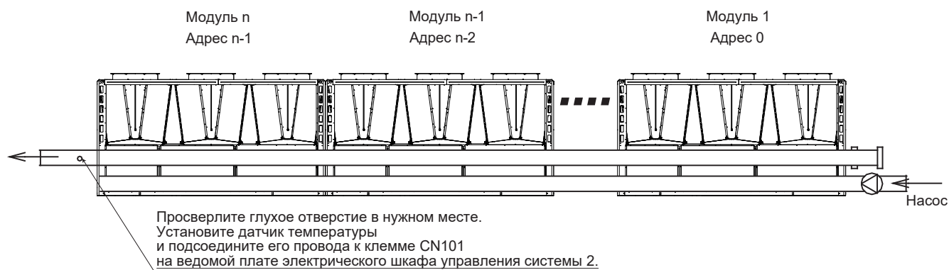
Рисунок 8-21. Установка нескольких модулей (не более 16)
