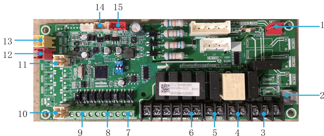
Рисунок 8-6. Ведомая плата
