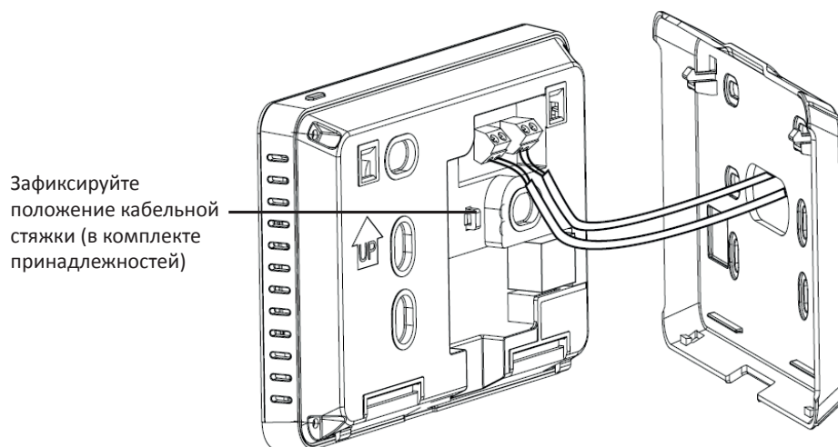
Рисунок 4 Схема подключения пульта ЦУ и отверстие для крепления кабельной стяжки
