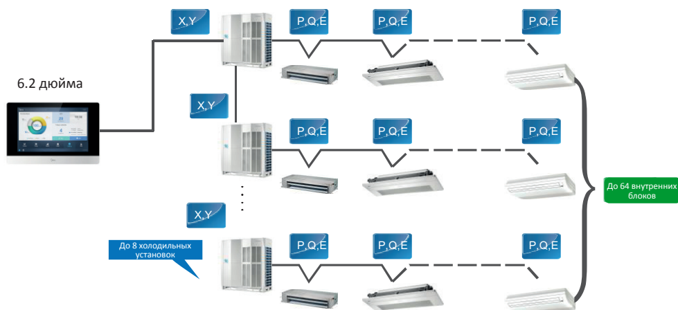
Рисунок 7(a) Соединение пульта ЦУ с наружными блоками
