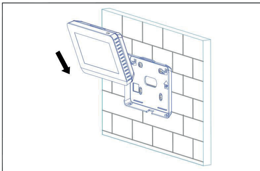
Рисунок 5 Вставьте пульт ЦУ в заднюю крышку
