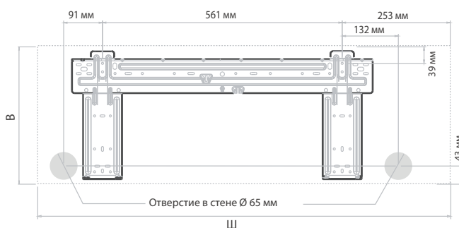
Размеры внутреннего блока (Ш×В): 968 x 322 мм
