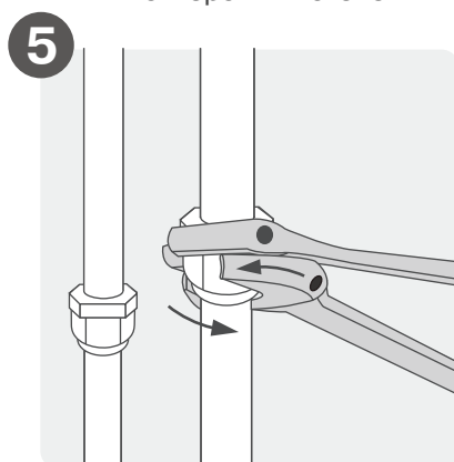
Соедините трубопроводы
