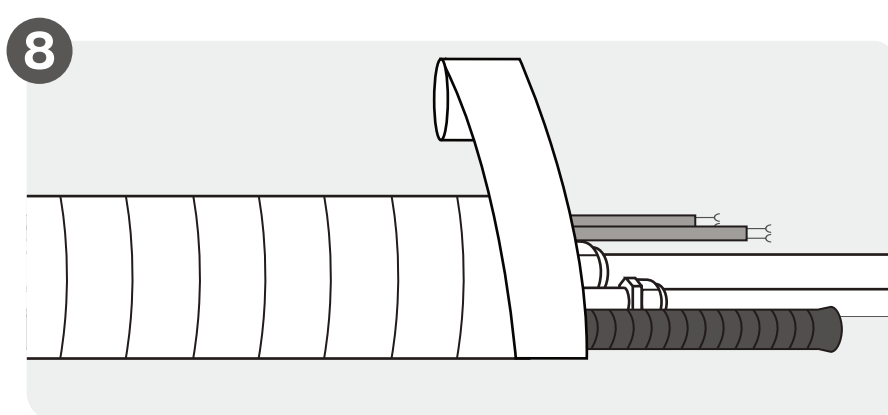
Обвяжите трубопроводы и кабели
