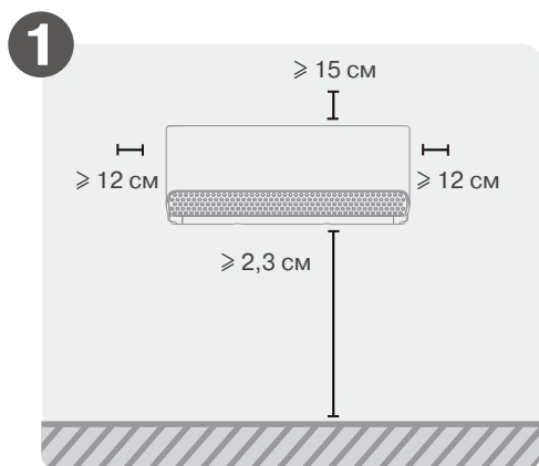
Выбор места для установки
