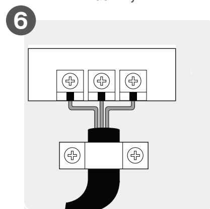
Подключение кабелей
