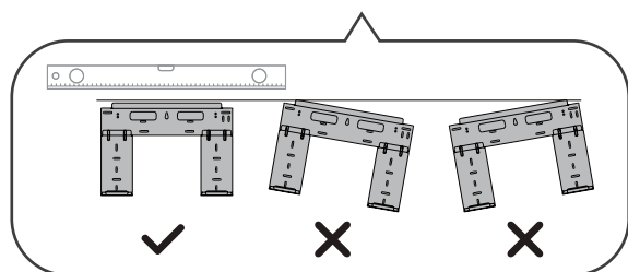
Правильное положение монтажной пластины
