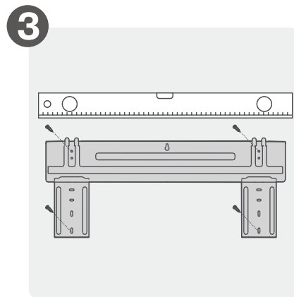
Закрепите монтажную пластину
