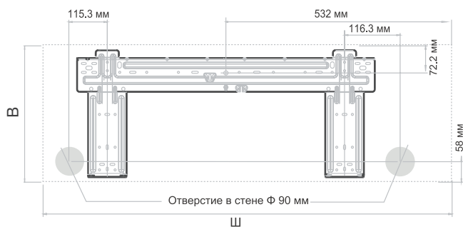
Размеры внутреннего блока (Ш×В): 1030 x 338 мм
