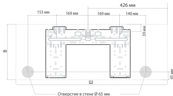
Размеры внутреннего блока (Ш×В): 812 x 299 мм
